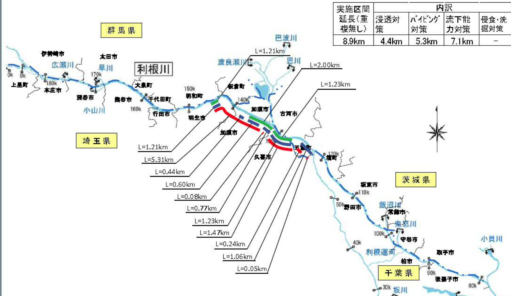
洪水を安全に流すためのハード対策 概要図 <利根川上流>
