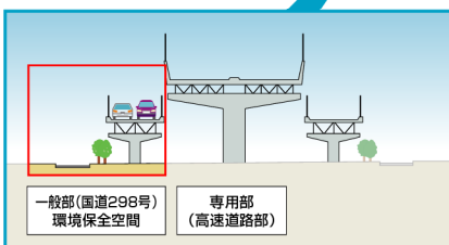
矢切高架橋(A断面)
