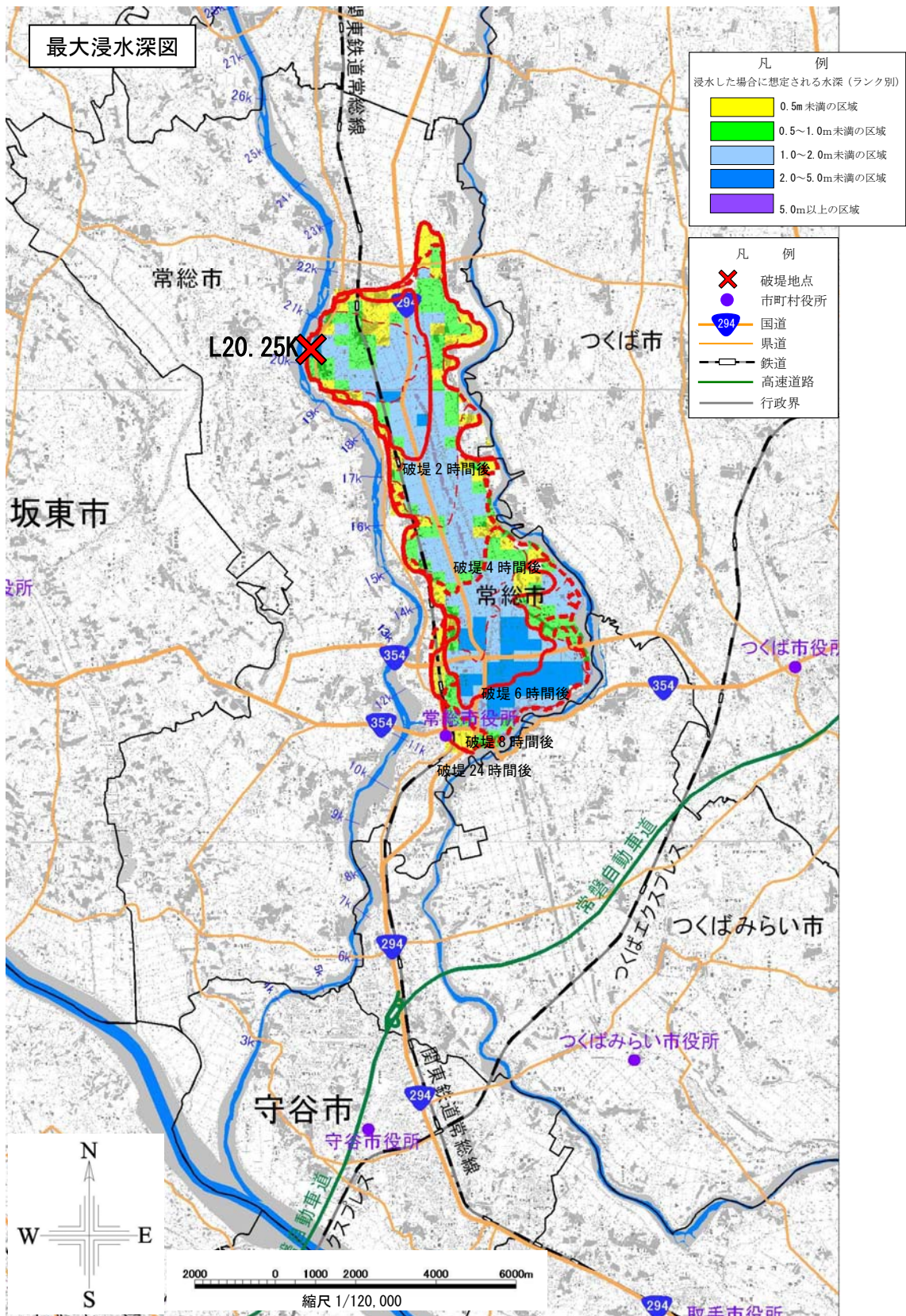
氾濫発生情報図 鬼怒川 左岸 20.25K
