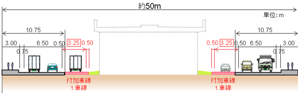
【計画断面図】
