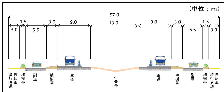
開通区間の標準断面図 (2/4車線)
