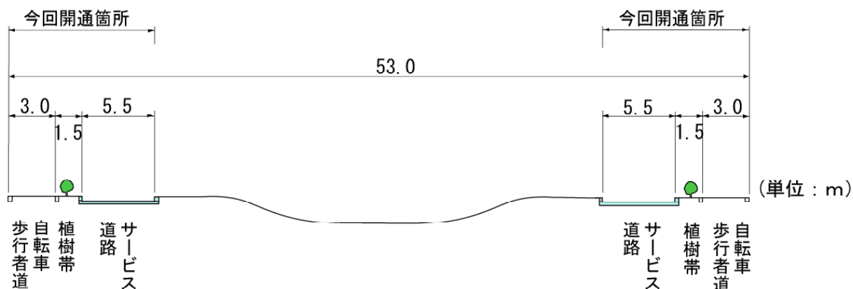
今回開通する区間の断面図
