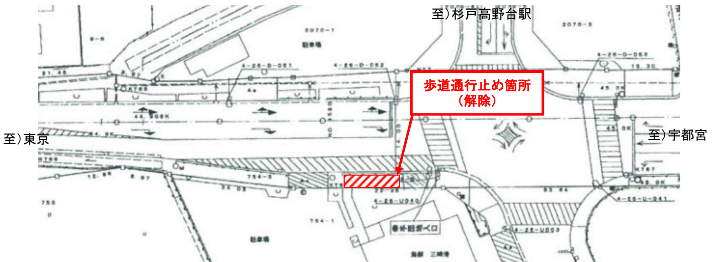
切り回し図
