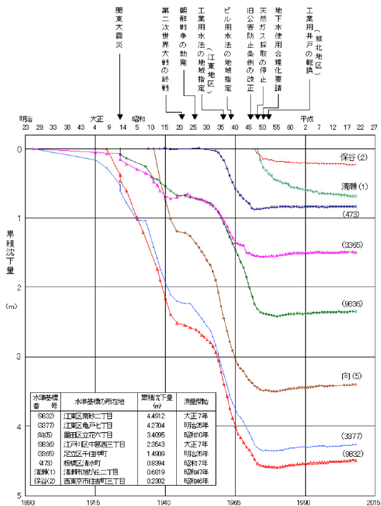
図 1-9 荒川下流部の主要水準基標の累計変動状況
