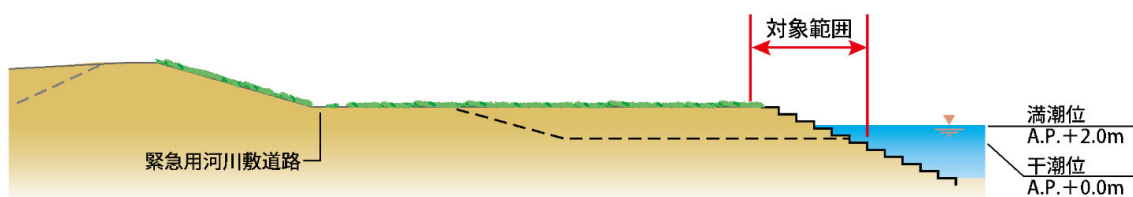
図 2-17 親水タイプの横断形状イメージ（例）
