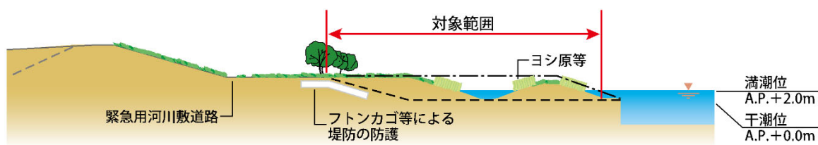
図 2-16 湿地化タイプの横断形状イメージ（例）
