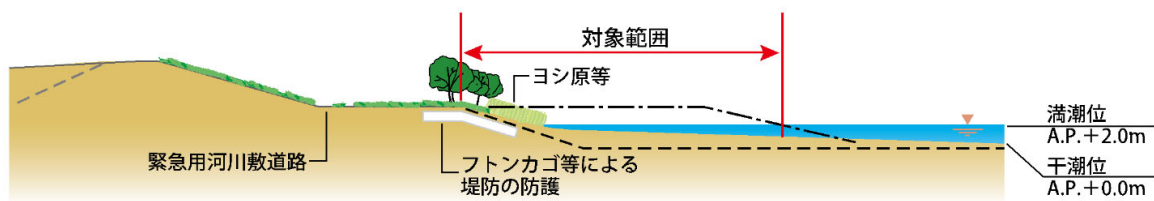
図 2-15 干潟タイプの横断形状イメージ（例）
