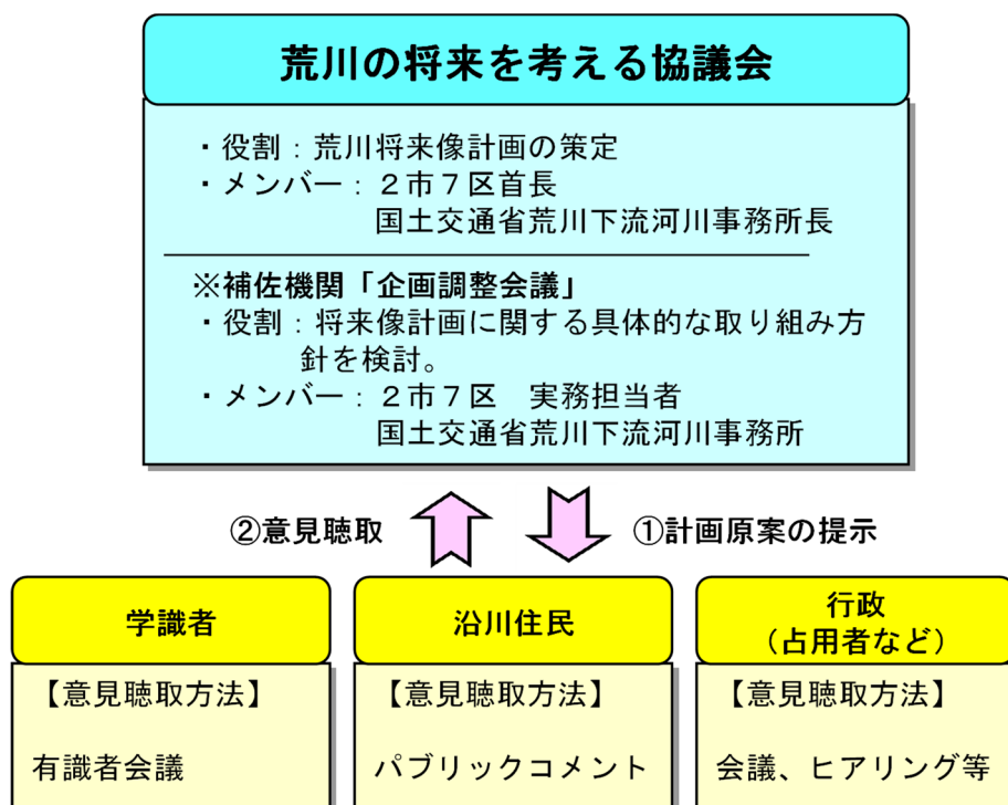
図 1-1 荒川将来像計画の検討体制
