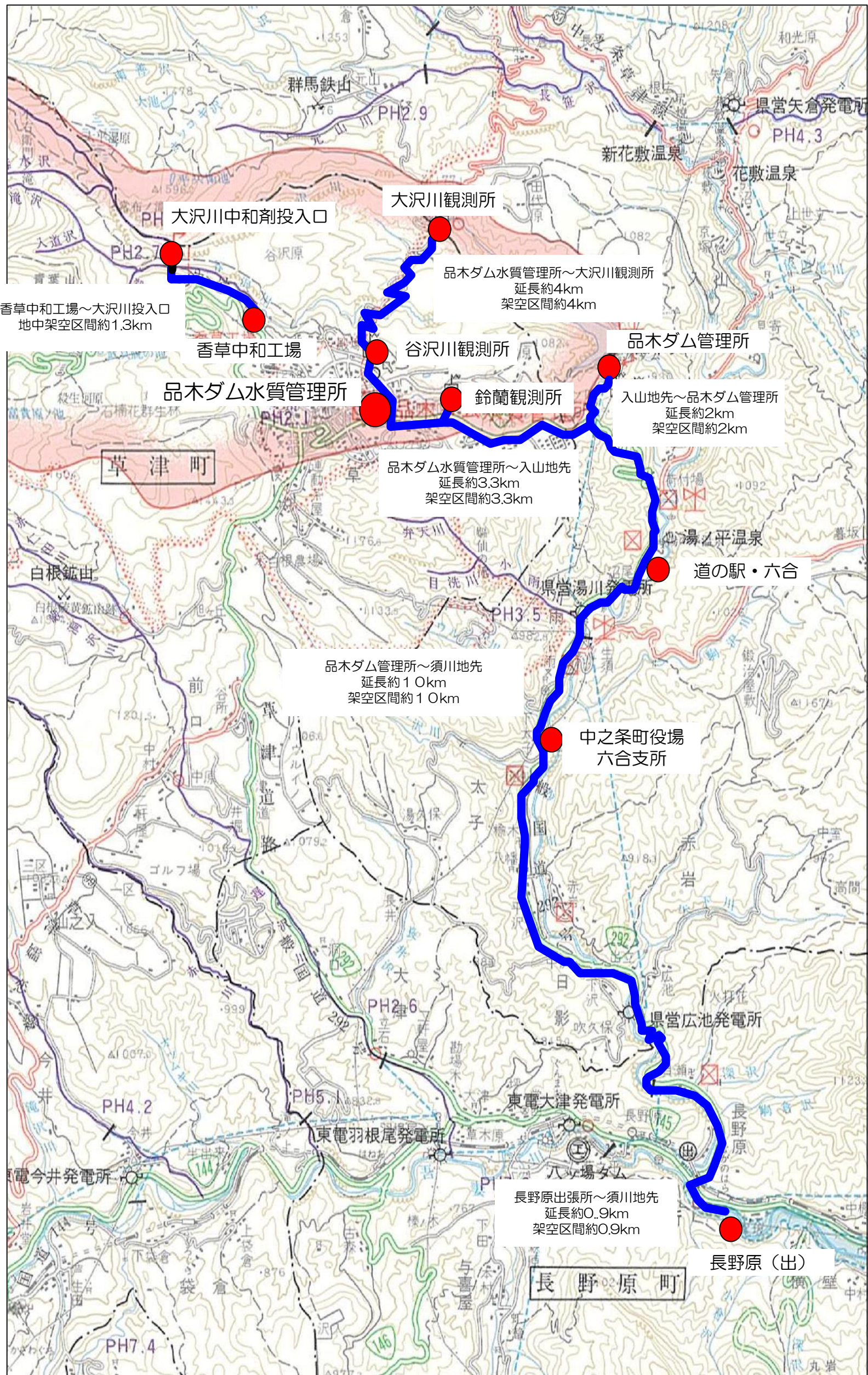
別図-1 品木ダム電気通信設備図
