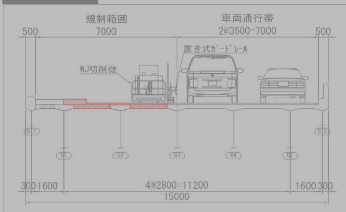
A-A断面図
