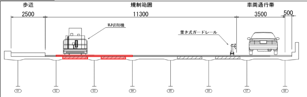
B-B断面図
