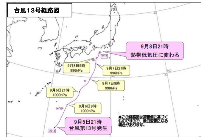
出典: 令和5年台風第13号に関する茨城県気象速報 (水戸地方気象台)
