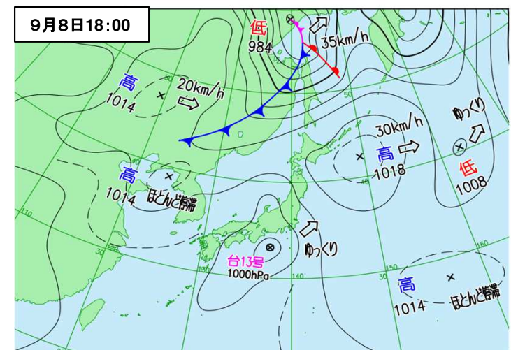
出典: 防災情報 9月8日18:00天気図 (気象庁)
