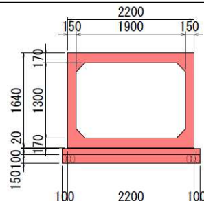
堤外水路（第三樋管側）標準断面図
