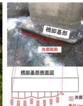
橋脚の洗掘
