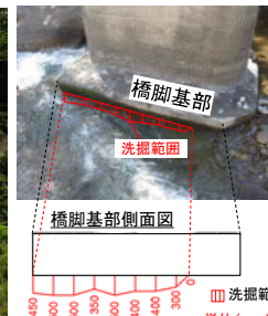
橋脚の洗掘
