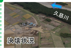
常陸大宮市塩原地区 久慈川左岸 27.0k付近
