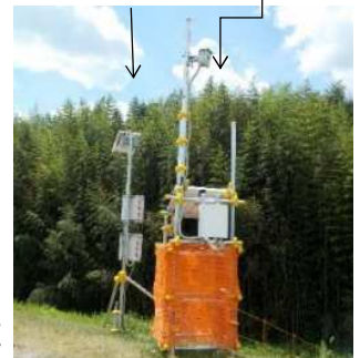
簡易型河川監視カメラ 危機管理型水位計
