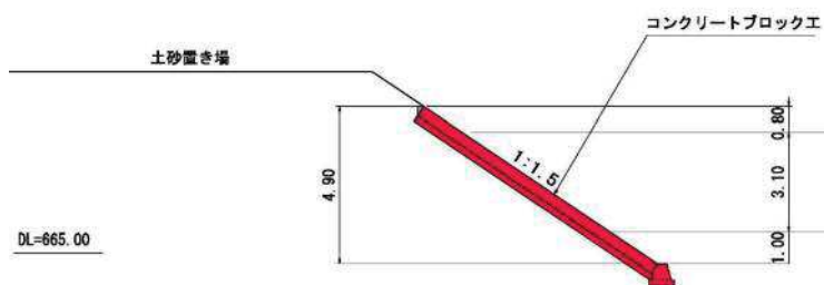
標準断面図
