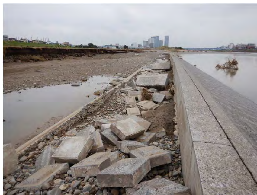
⑥多摩川 19.4k 左岸（東京都世田谷区） 低水護岸崩壊 L=91m
