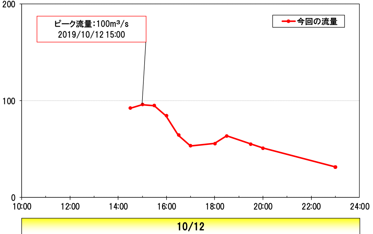
流量(m 3 /s) 高田橋流量観測所(早淵川1.4km 神奈川県横浜市港北区新吉田町)
