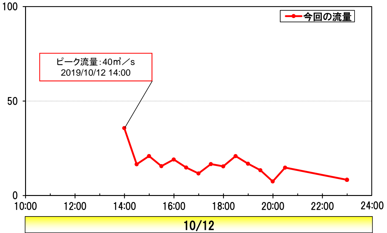
流量(m 3 /s) 鳥山流量観測所(鳥山川1.4km 神奈川県横浜市港北区鳥山町)
