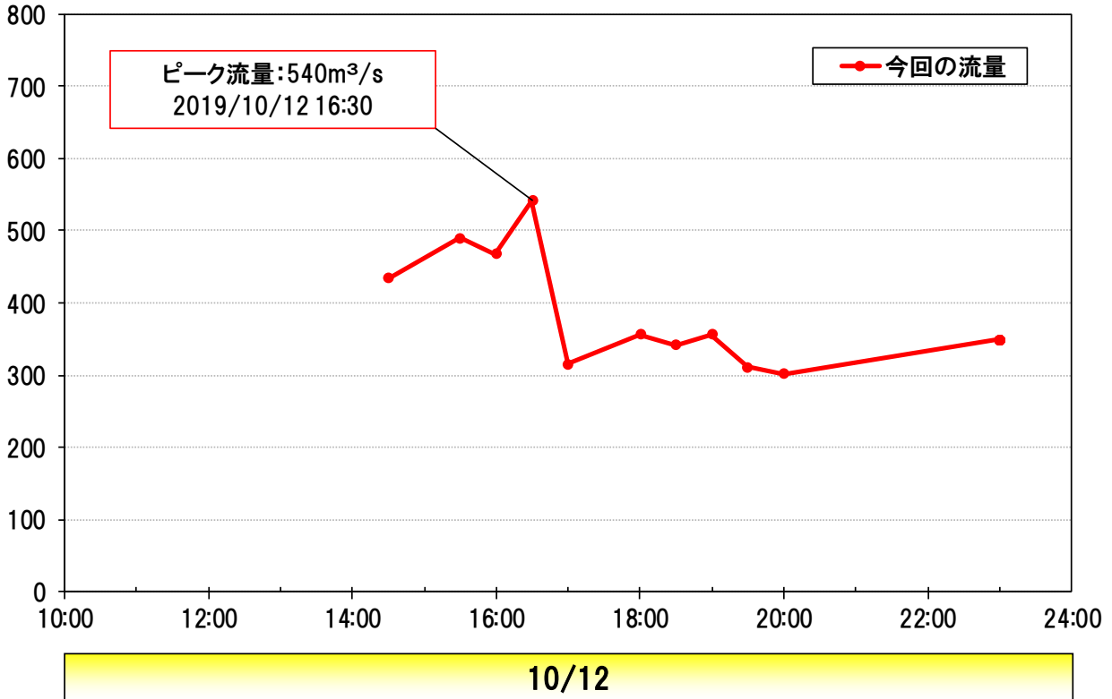
流量(m 3 /s) 太尾流量観測所(鶴見川10.8km 神奈川県横浜市港北区新羽町)
