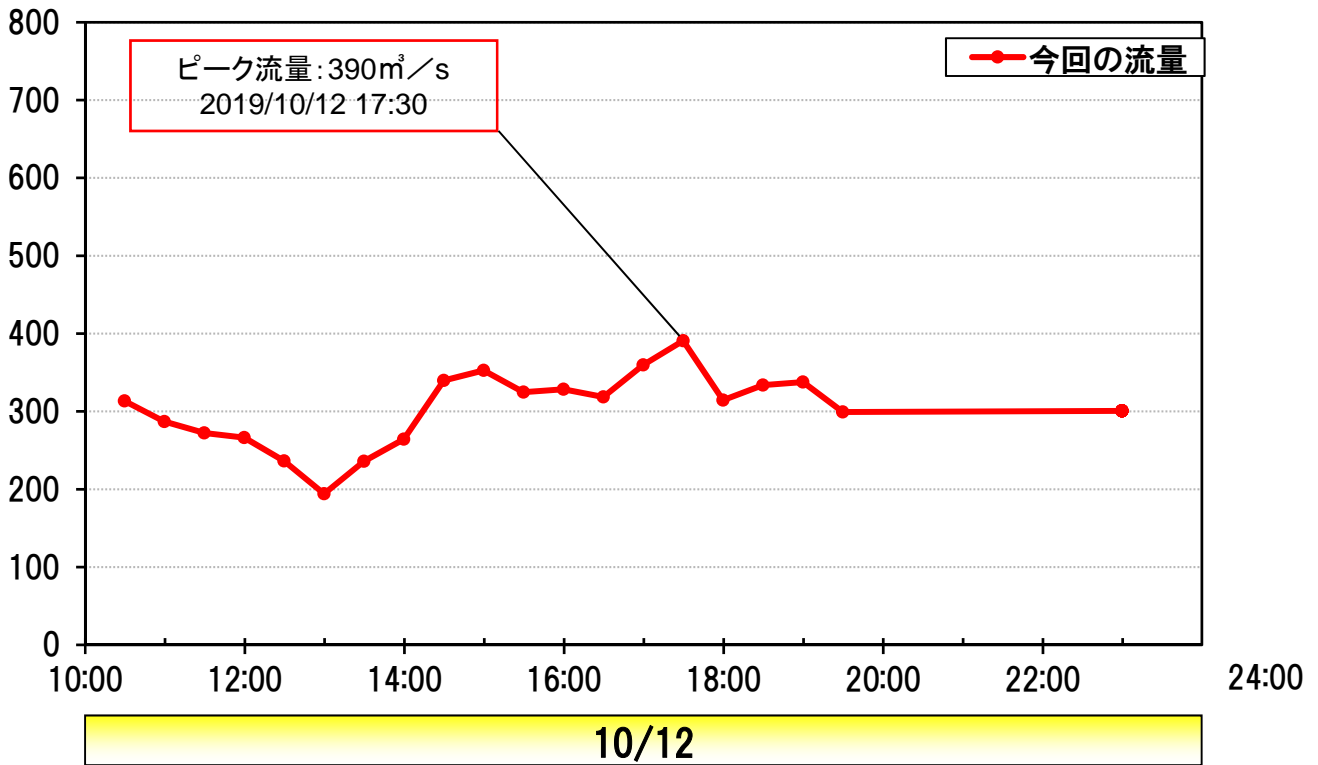
流量(m 3 /s) 亀の子橋流量観測所(13.8km 神奈川県横浜市港北区小机町)
