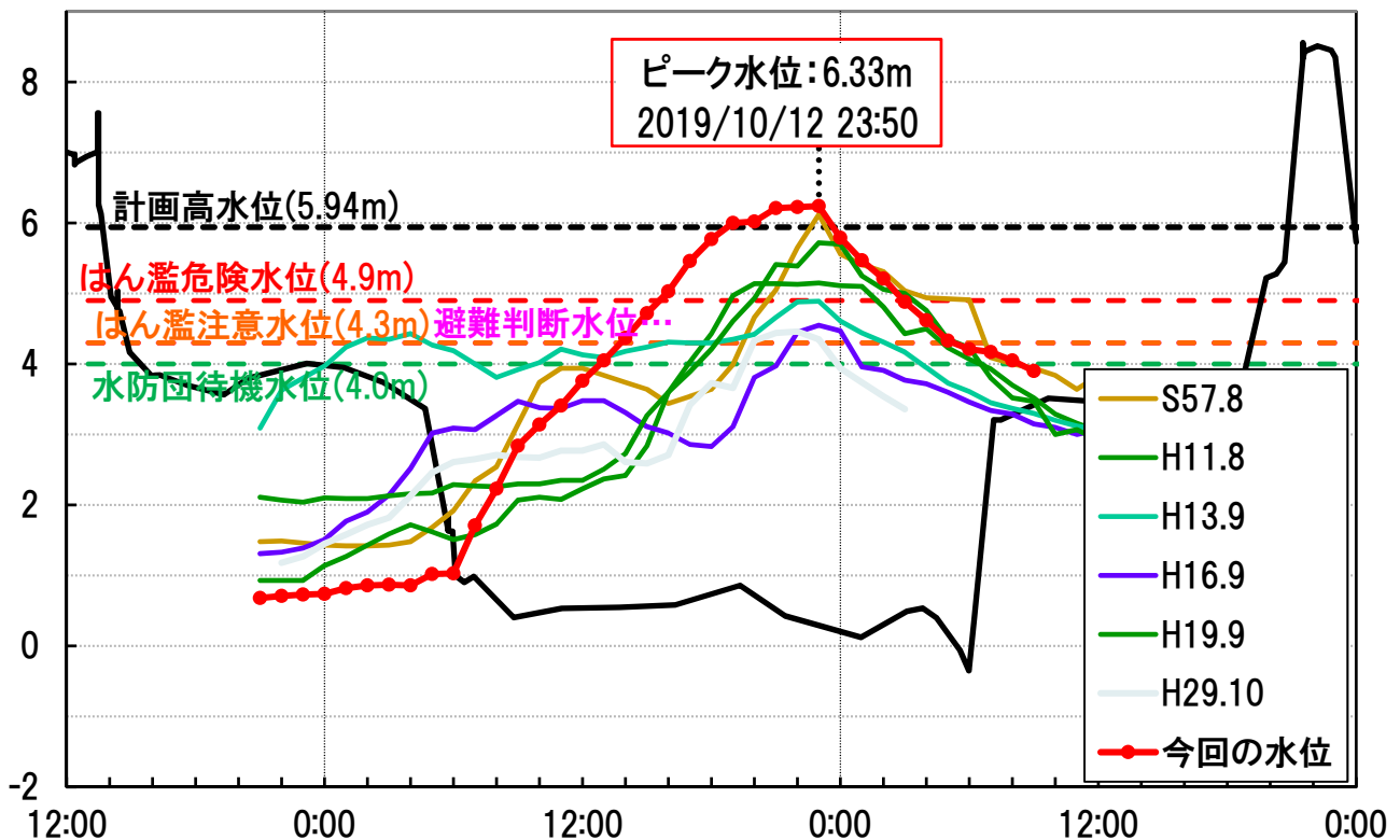
水位(m) 石原水位観測所(27.6k 調布市多摩川3丁目)
