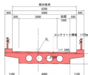
断面図 S=1:50
