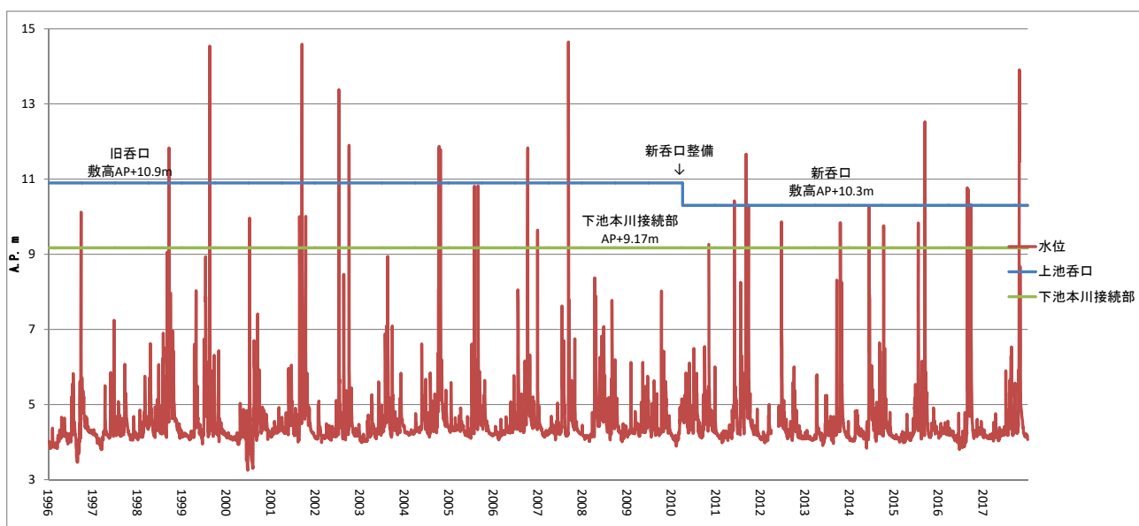
図 1-12 太郎右衛門橋水位観測所での日水位変化 平成 8～29 年(1996～2017 年)
