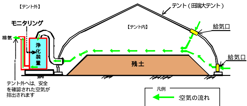
テント断面イメージ（残土仮置き場：田端大テント）
