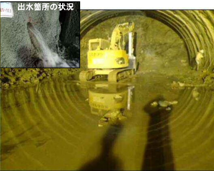
■トンネル坑内の冠水の状況(上八木沢トンネル) かみやぎさわ
