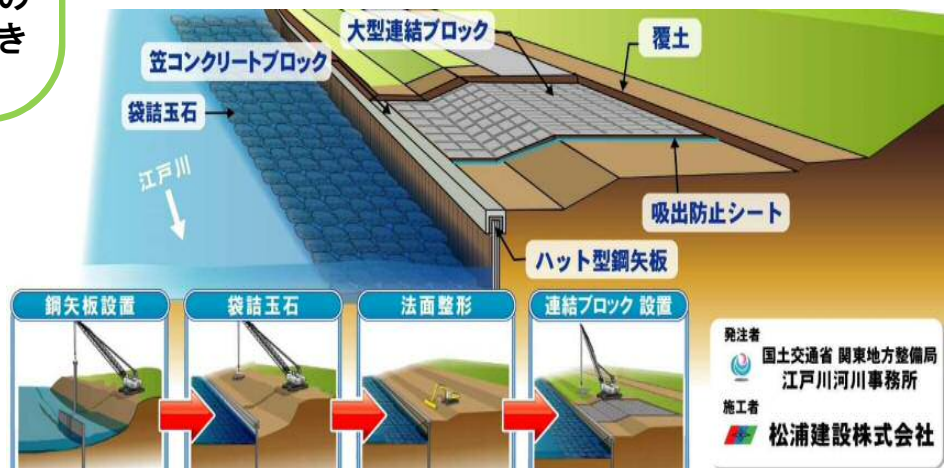
鋼矢板設置
