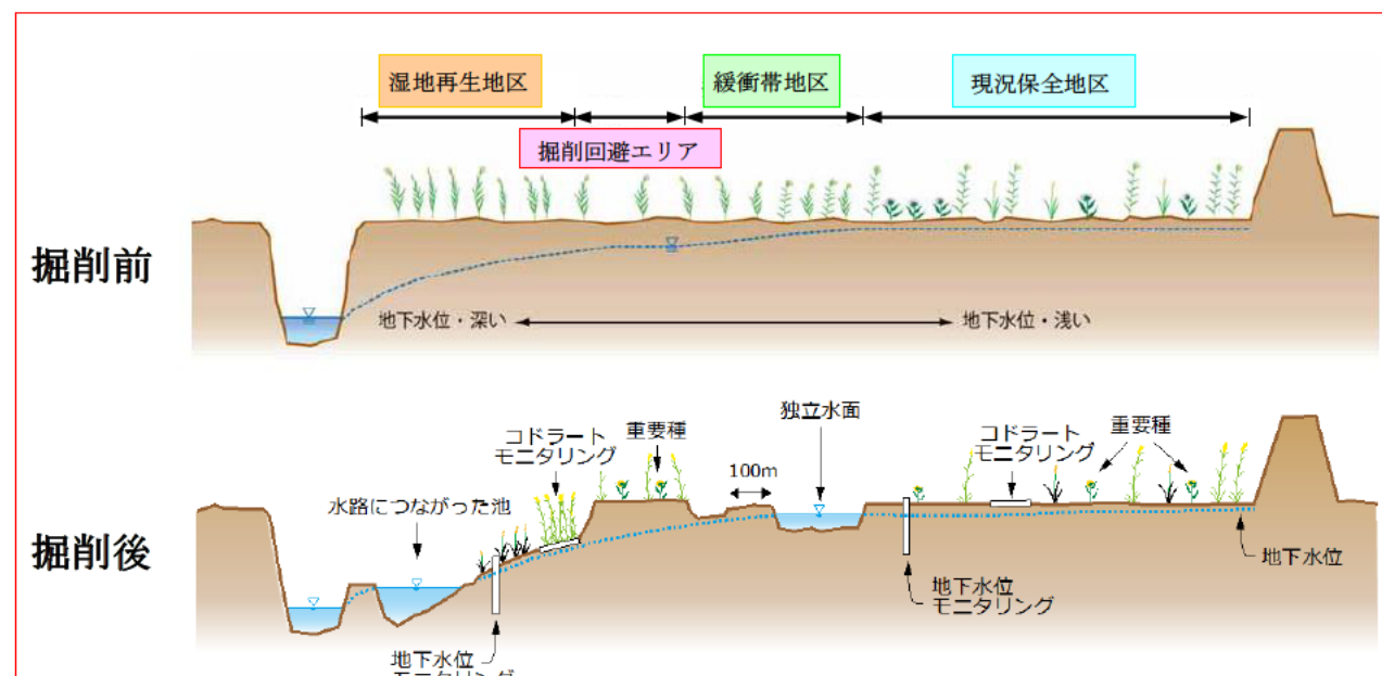
図 3-2 第 2 調節池のゾーニングの考え方 (横断面の概念図)
