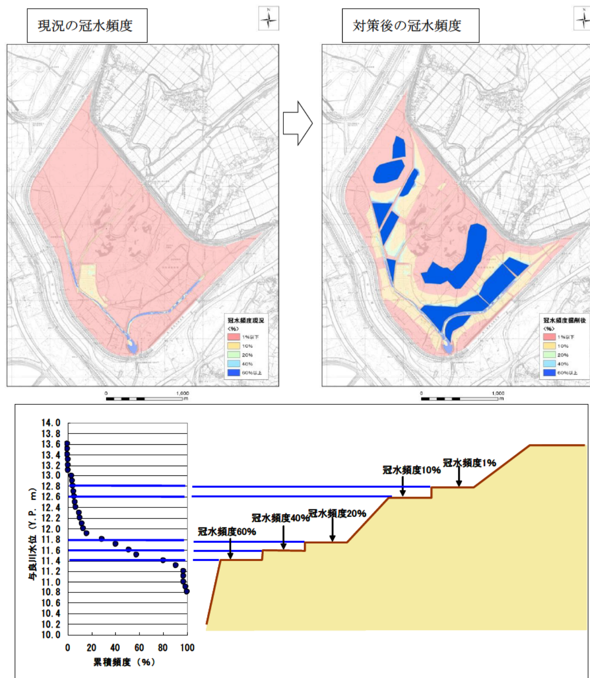
図3-10 掘削による冠水頻度の面的変化
