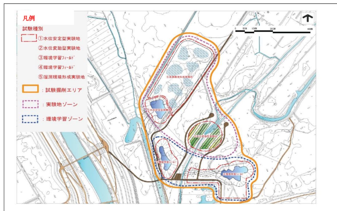
図4-4 試験施工エリアのレイアウト
