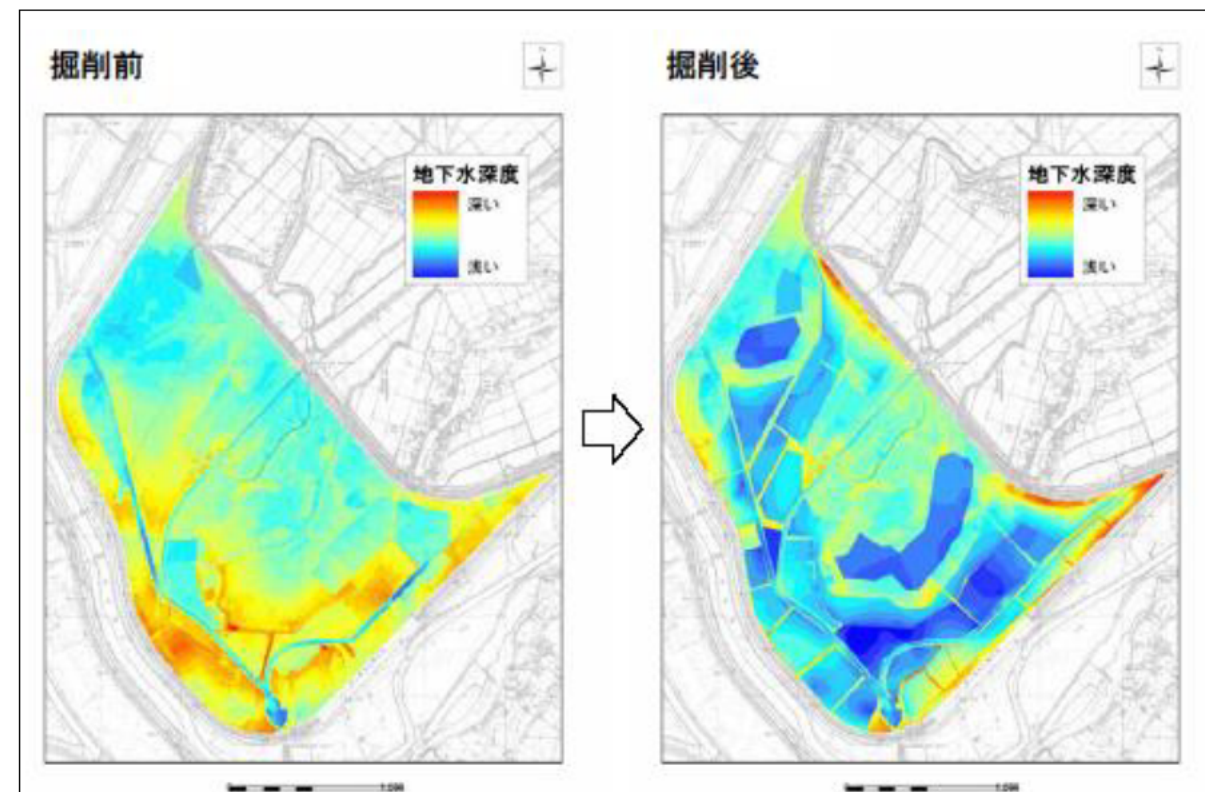
図3-6 地下水位分布の面的変化
