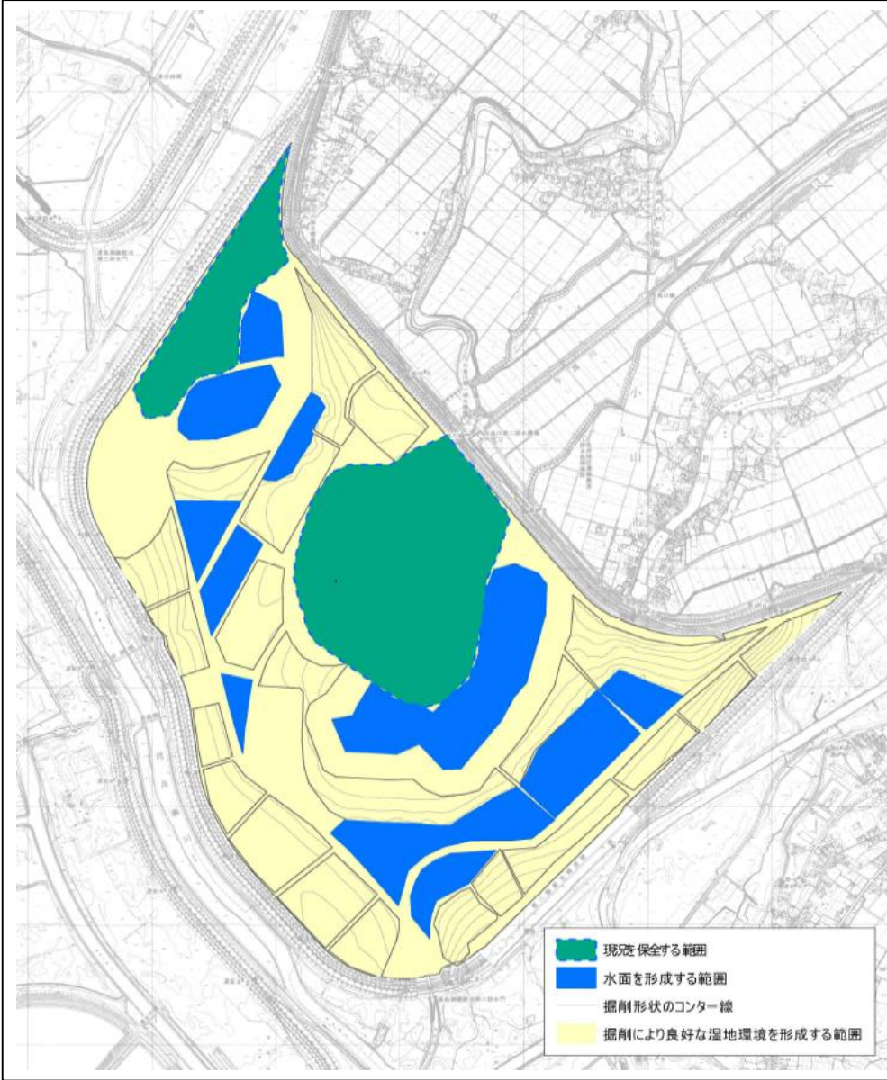
図 3-5 掘削計画図
