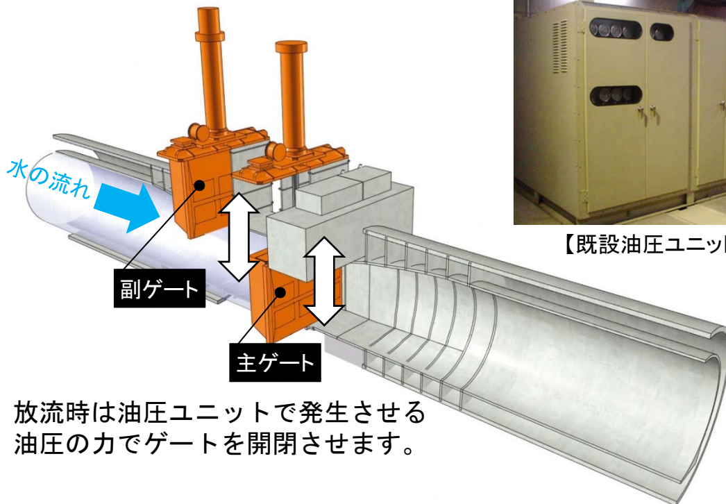
【高位常用洪水吐イメージ図】
