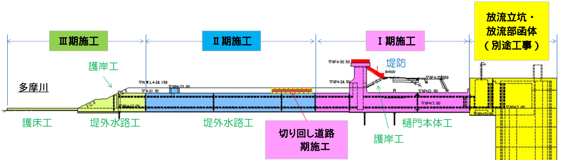
標準横断面図
