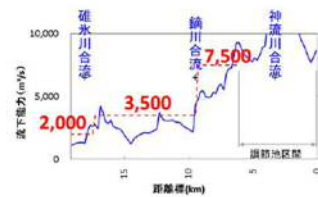
図 4-3 利根川の河道目標流量
