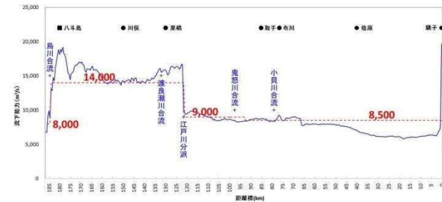
図 4-1 利根川の河道目標流量
