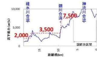
図 4-3 利根川の河道目標流量
