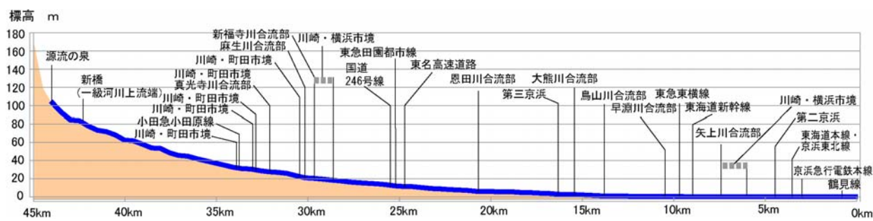
図 2.1.4 鶴見川本川の河川縦断面図
