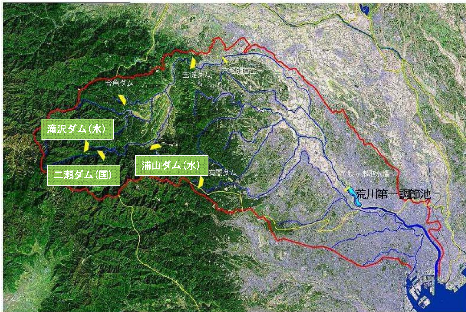
荒川水系における洪水調節施設
