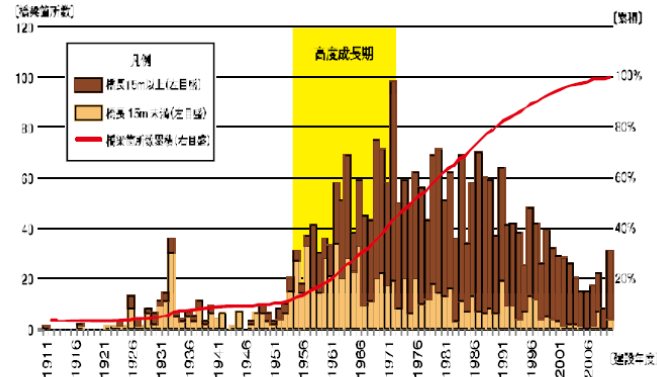
建設年度別の橋梁箇所数の分布
