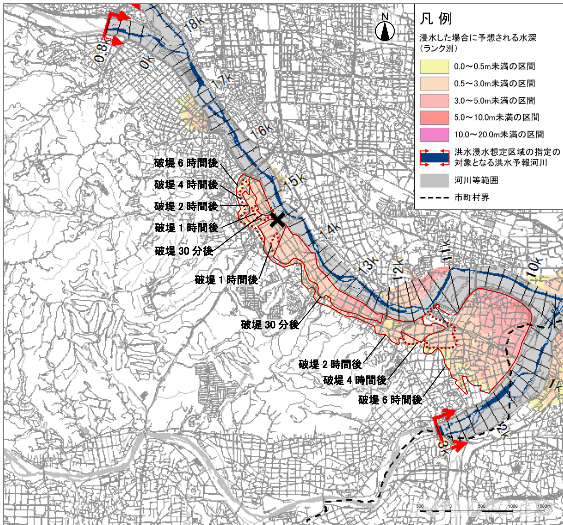
破堤箇所 烏川 右岸 14.6k
