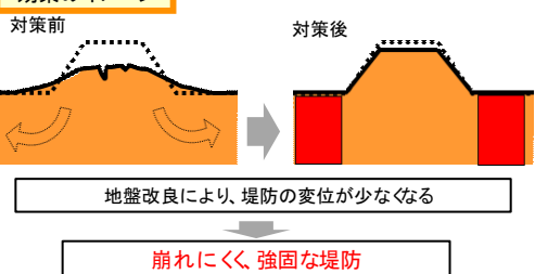
▲堤防強化対策（地盤改良）イメージ
