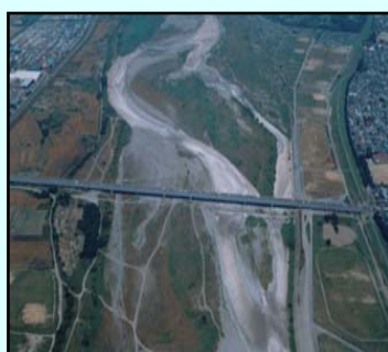
▲荒川大橋付近の瀬切(平成4年)
