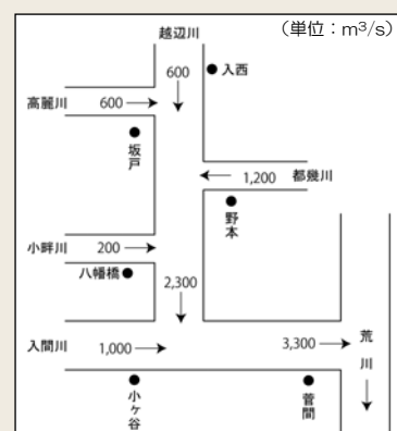
▲入間川整備計画流量図
