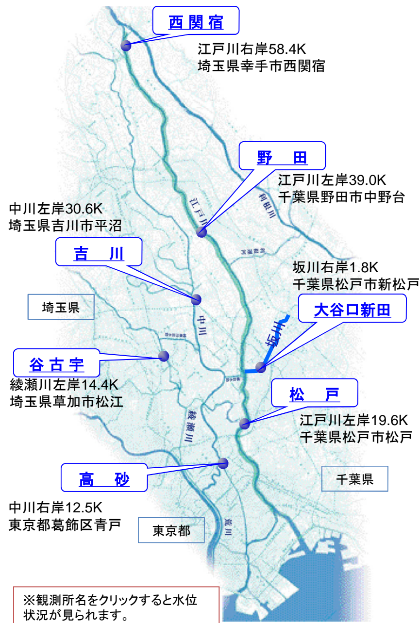
水位観測所位置図
