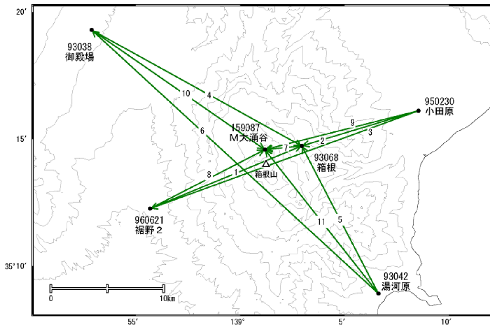
箱根山周辺 GNSS連続観測基線図
