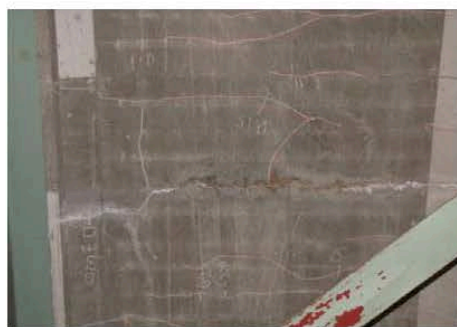
床版のひびわれ及び遊離石灰の析出状況
