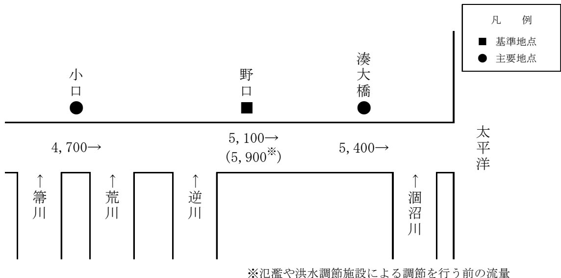
図 4-1 那珂川流量配分図
