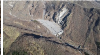
国内有数の大規模堰堤「日向砂防堰堤」（S3完成、S57改築）
