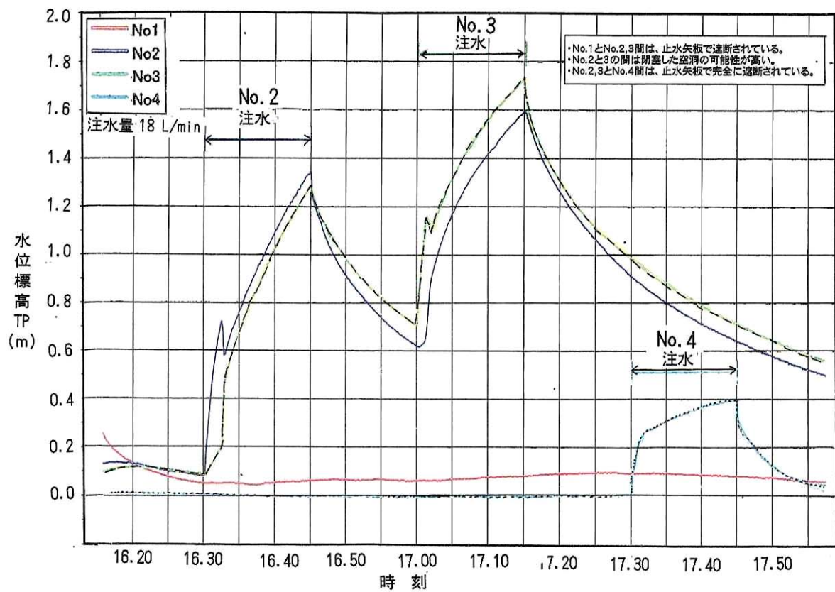
図-28 連通試験結果 事例3 (C樋門)
