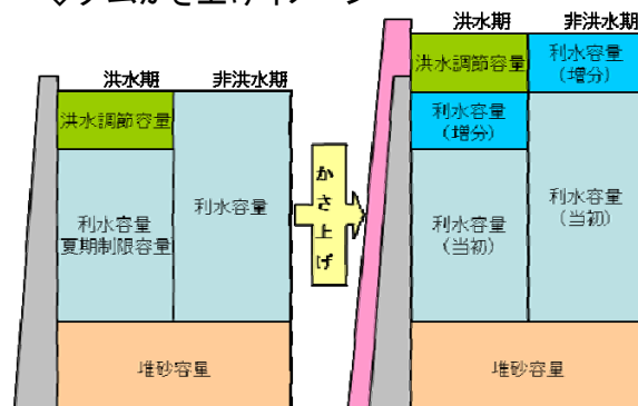
図 4.4-33 かさ上げイメージ図
