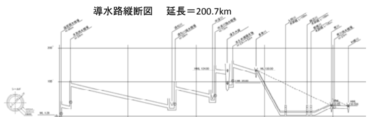
図 4.4-15 導水路縦断面図
