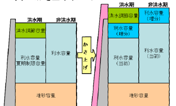
図 4.4-33 かさ上げイメージ図
