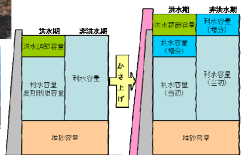
図 4.4-9 かさ上げイメージ図
