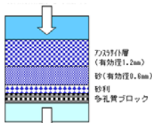
出典：土浦市ホームページ 急速ろ過法 http://www.city.tsuchiura.lg.jp/index.php?code=501
