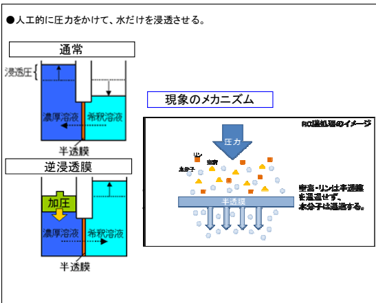
出典：近畿経済産業局 海水淡水化用逆浸透膜エレメント http://www.kansai.meti.go.jp/team_e_kansai/member/tech/nittou.pdf
