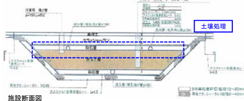
施設断面図
