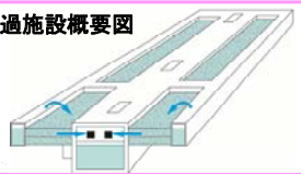
■砂ろ過施設概要図
