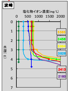
図3 塩化物イオン濃度の鉛直方向の分布(常陸川水門~6K)
