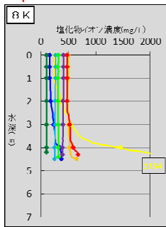
図2 塩化物濃度イオンの鉛直方向の分布(常陸利根川 7K~12K)
