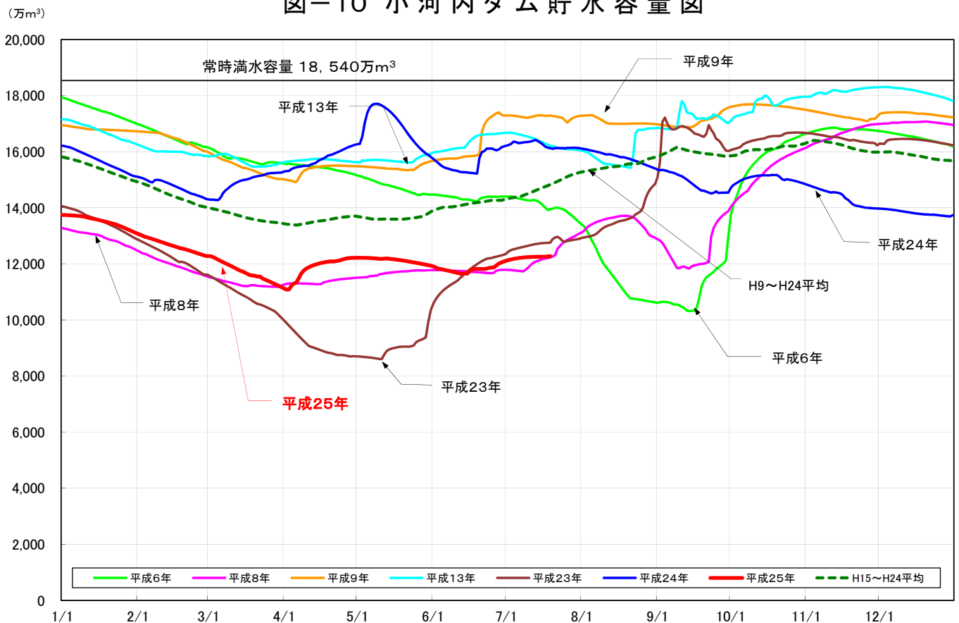
図-10 小河内ダム貯水容量図
