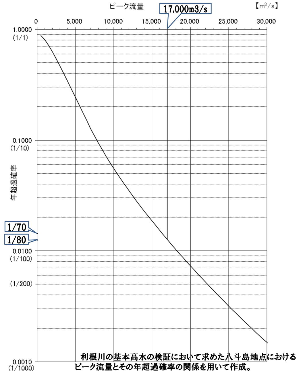
図 八斗島地点におけるピーク流量－年超過確率
