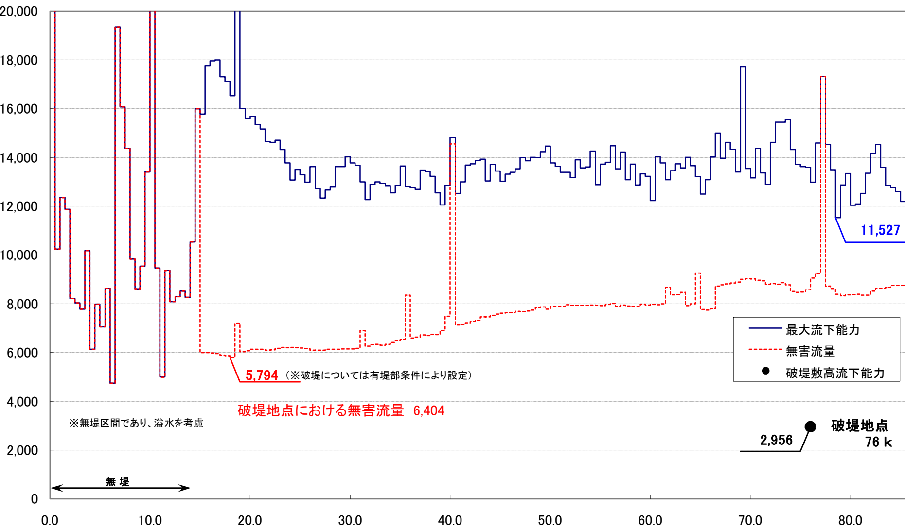
様式-3 氾濫ブロックG 流下能力図
