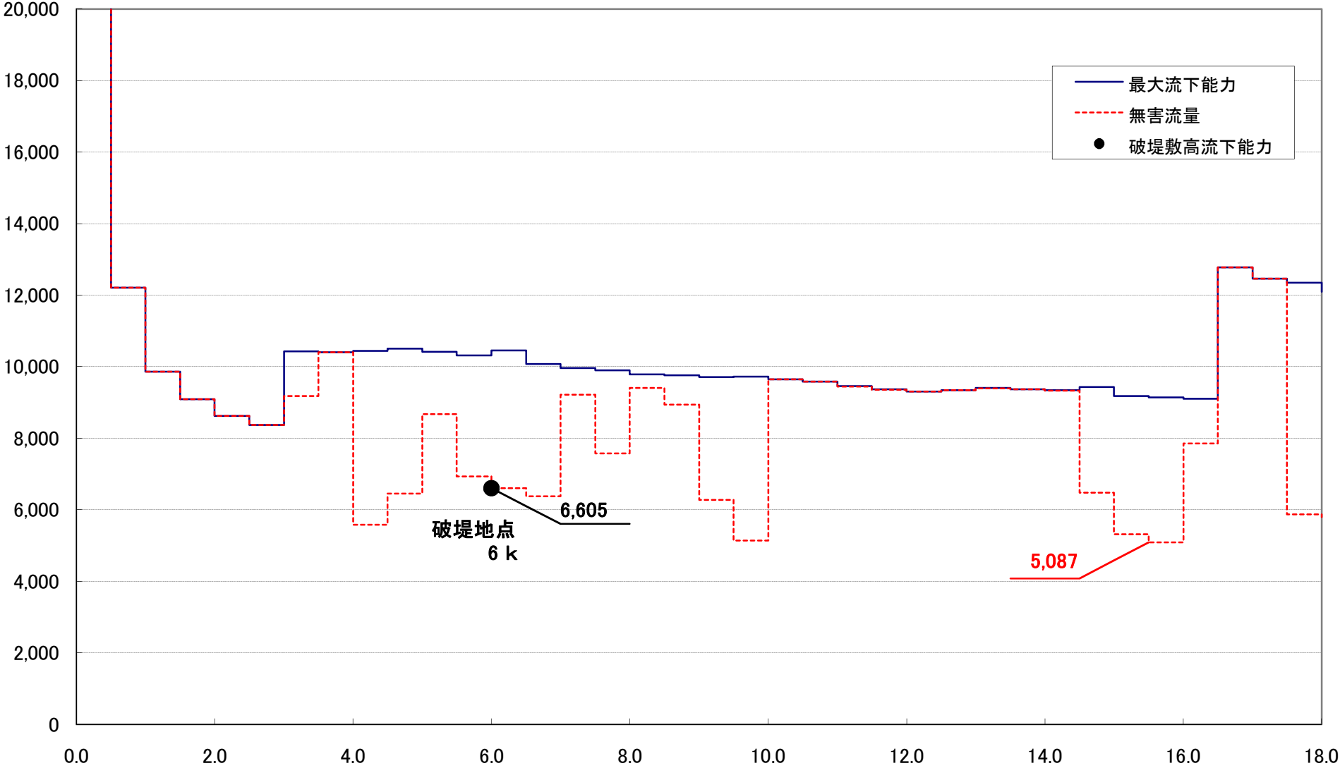
様式-3 流下能力図 氾濫ブロックD-2
