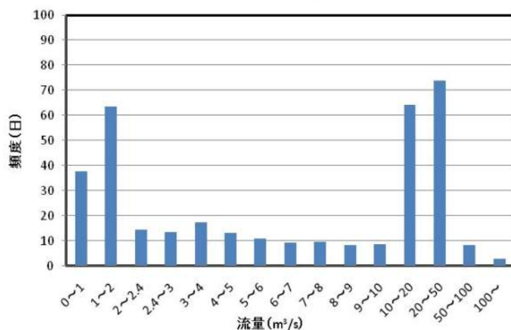
吾妻峡に流れる流量とその頻度
