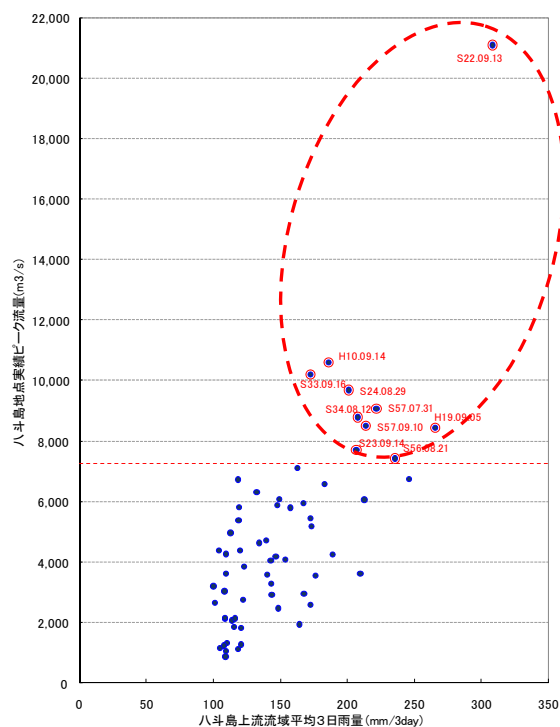
八斗島上流における流域平均3日雨量と実績流量の関係
