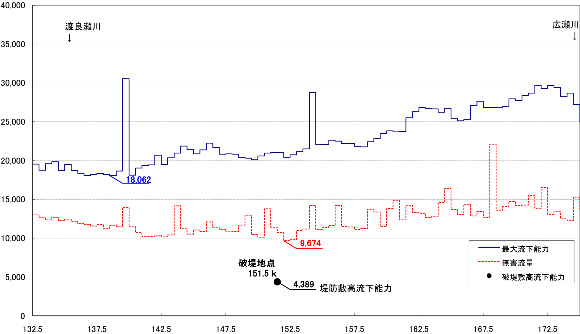
様式-3 氾濫ブロックA
