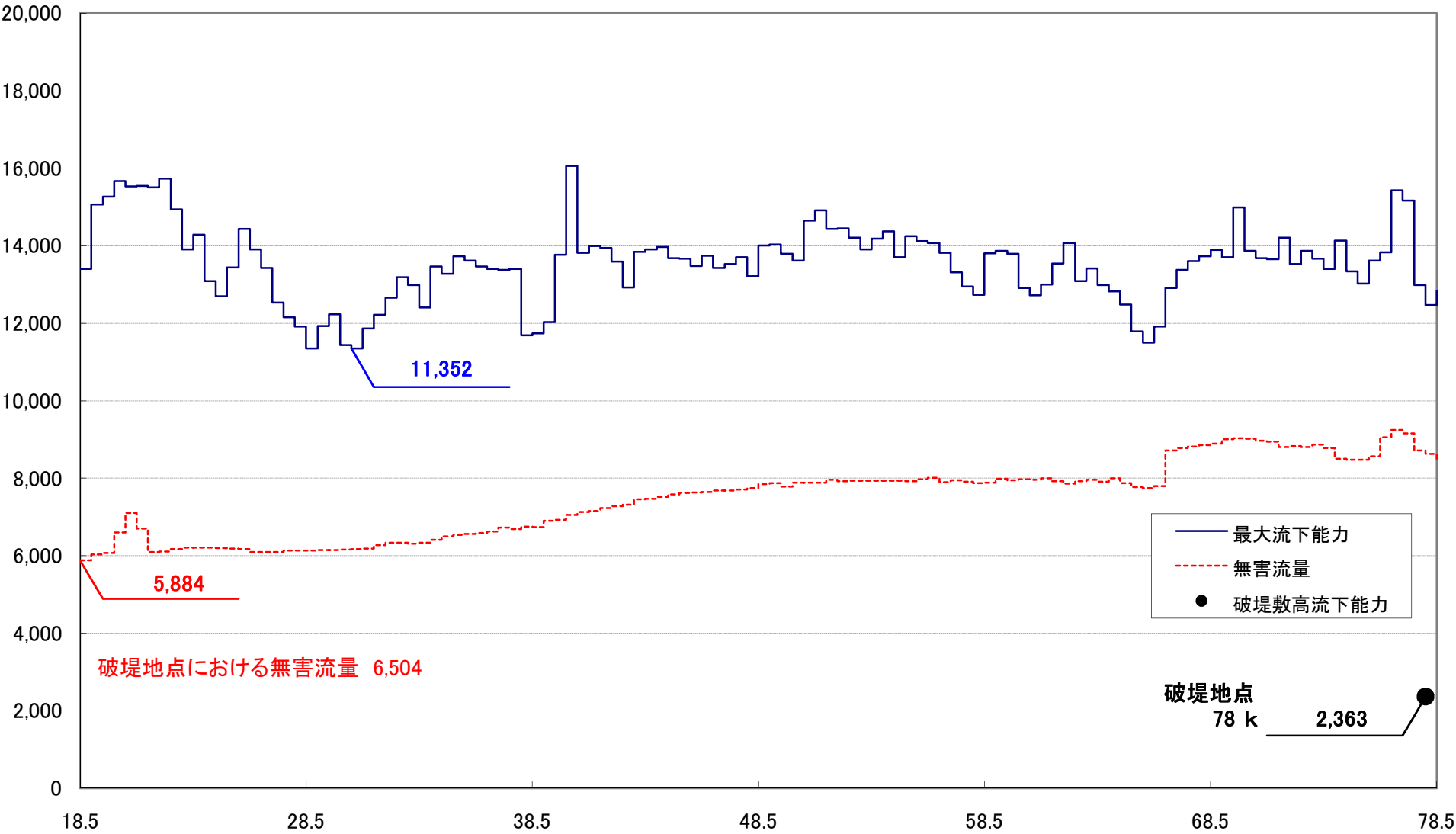
様式-3 流下能力図 氾濫ブロックD-1
