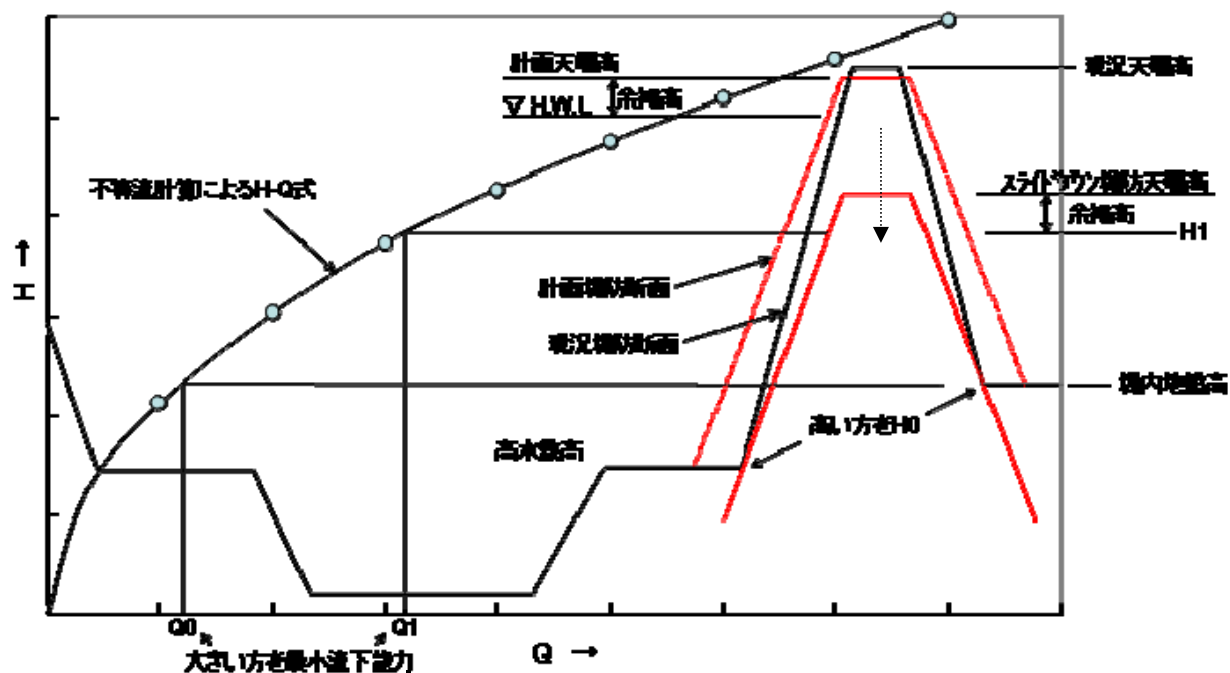
最小濾下能力の設定イメージ
