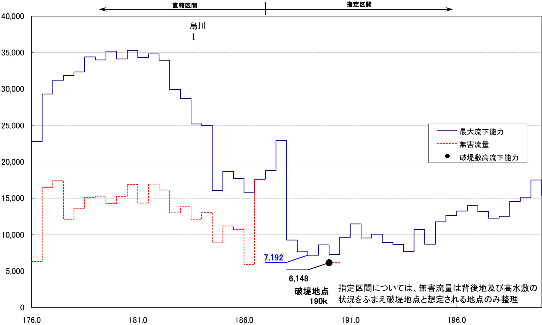
様式-3 氾濫ブロックH
