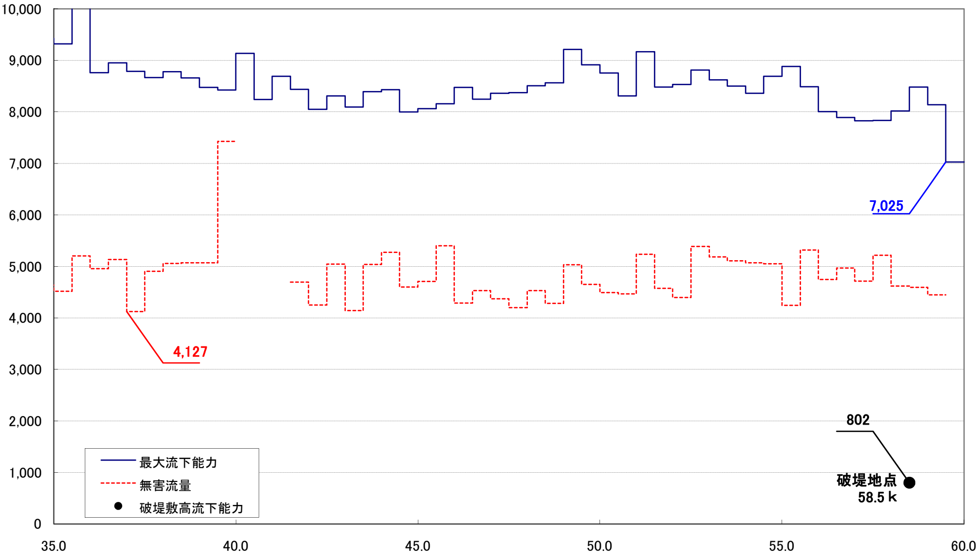
様式-3 流下能力図 氾濫ブロックF3
