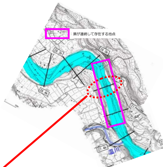
図 4-4-3 瀬の平面図
