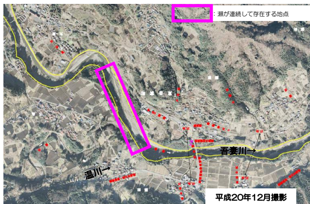
図 4-4-3 瀬の平面図
