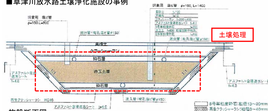
施設断面図
