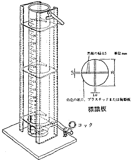
透視度計
