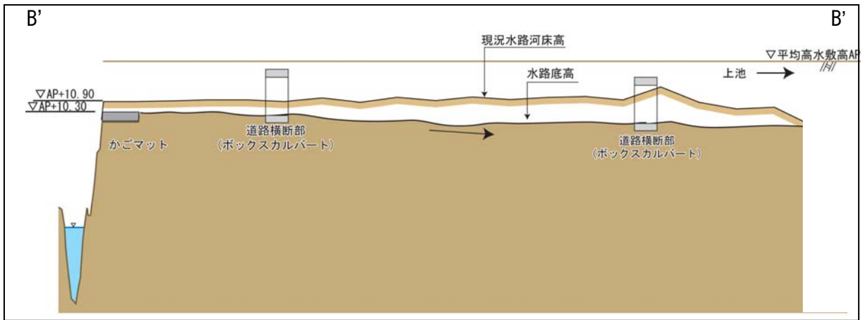
図 2-25 呑口付近縦断面図
